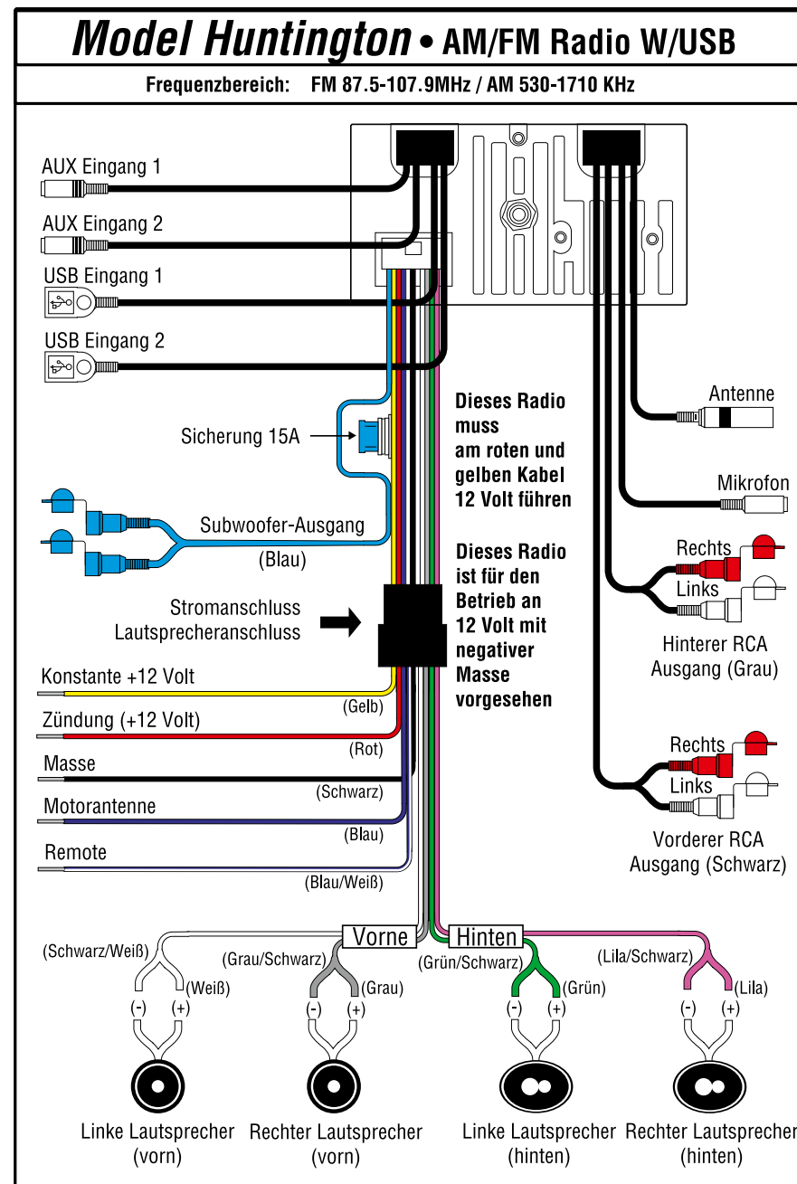
Abbildung 8 - Kabelplan
